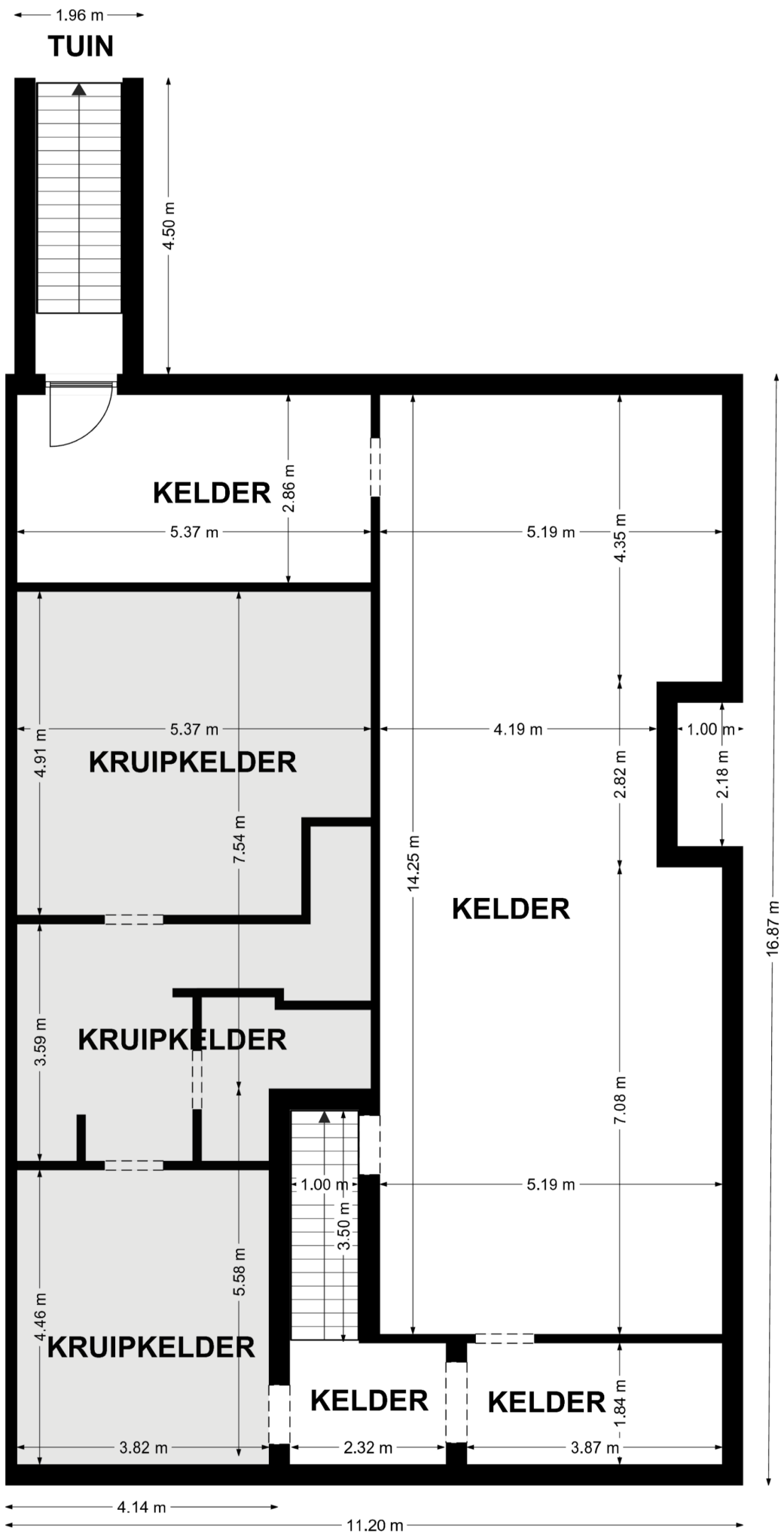
Steenkuilstraat 86 schets kelderverdieping maten zijn bij benadering
